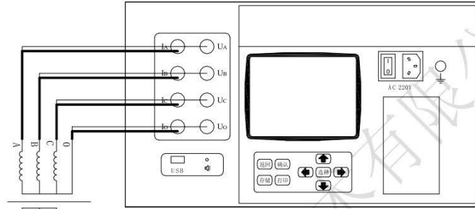
高压侧三相、单相、单线测试接线图
