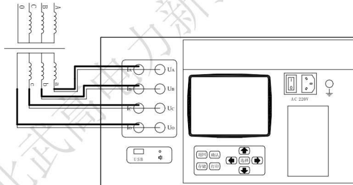
低压侧三相、单相、单线测试接线图
