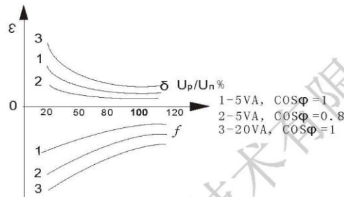
电压互感器电压与负荷特性
