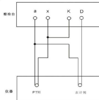
PT 二次压降检定接线图
