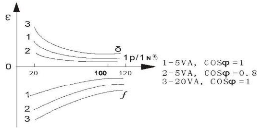
电流互感器的负荷特性曲线
